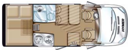
Hymer Fahrzeugmaße: LxHxB: 5,98 x 2,72 x 2,14 m
